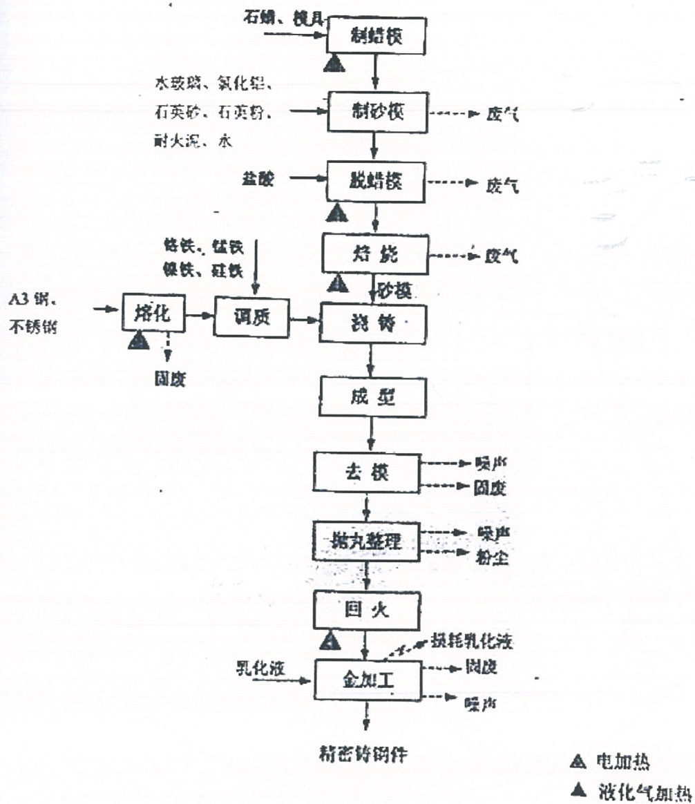
图 1 工艺流程图
